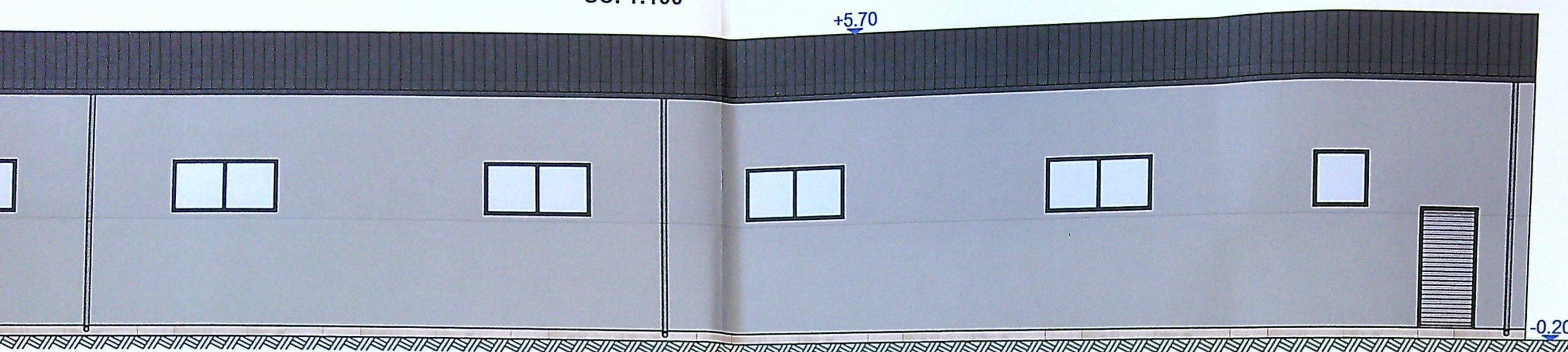
FAȚADĂ PRINCIPALĂ SC. 1:100
