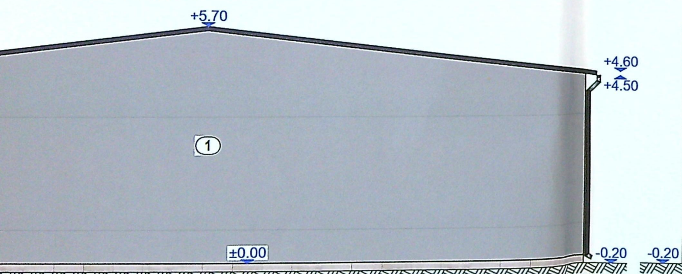
FAȚADĂ LAT. DREAPTĂ SC. 1:100
